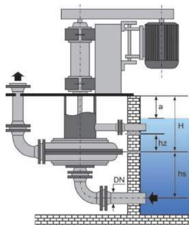
Сухая установка V310
