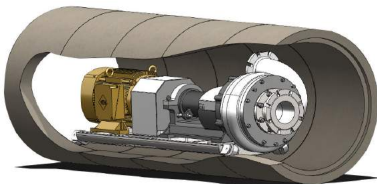
КВ 100 в микротоннелировании – диаметр 700 мм
