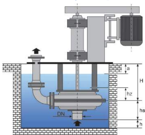
Погружная установка V300 ( H_s = макс. 2500 мм)
