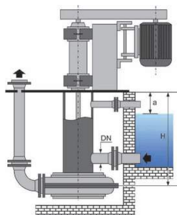
Сухая установка V330
