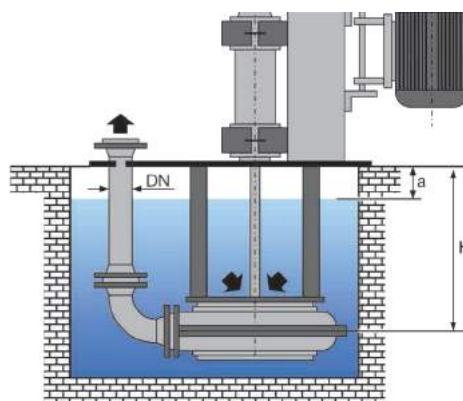
Погружная установка V320 / V340 (V340 с дополнительным всасывающим патрубком снизу)
